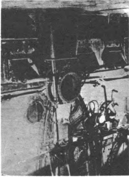
KAZAN DAİRESİ — Göeben (Yavuz) 136 ocaklı ve 24 kazanlıydı.
