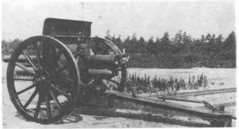
Rus topu : 76.2 - mm M—1903
