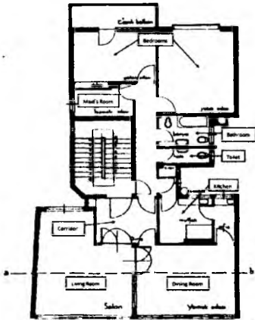
RESİM 4. Bayan Firdevs Evi, Seyhanlı Apartmanı, kat planı, Maçka. Mimar: Sedat Hakkı Eldem (Arkitekt, 12, 48, 1934, s. 334).
