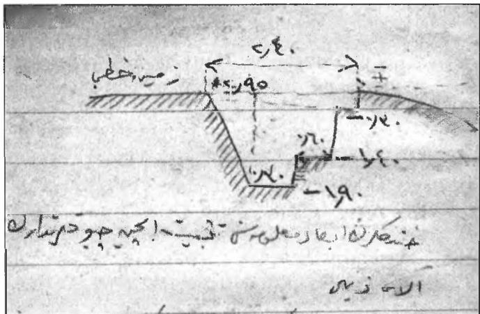
Avcı hendeklerinin ölçülerinin verildiği çizim
