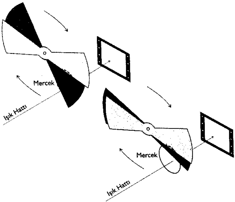
Resim 2-20. DEĞİŞİR ÖRTÜCÜ. Fotoğrafta örtücü (obtüratör) yalnızca yaylı metal plaka ya da bez bir perdedir. Ancak sinemada pozlama süresi saniyede 24 kare standart hızla sınırlıdır. Değişir örtücü, pozlama süresinde esneklik sağlar. Her ne kadar yine saniyede 24 kare hızla dönmeye de deliğin büyüklüğü ve bundan dolayı da pozlama süresi üst üste binen plakaları düzenleyerek değiştirilebilir.
