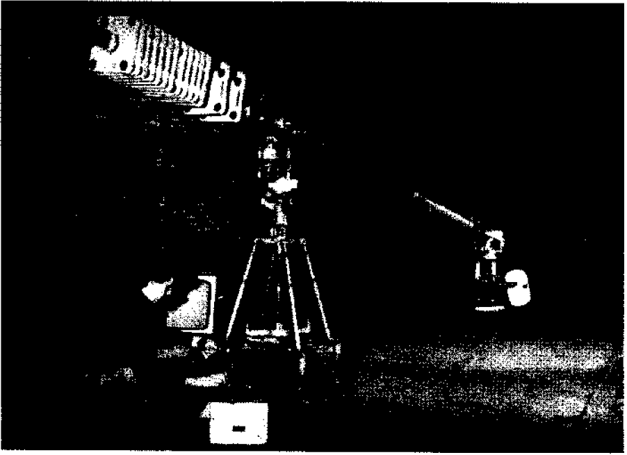
Resim 2-31. LOUMA VINCI. Görüntü yönetmeni televizyon monitöründen kameranın çektiği görüntüyü izlerken servo-motorlarla vinci ve kameranın hareketini kontrol eder. Vincin çok ani yön değiştirme kapasitesi vardır. Kameraya takılan bir zoom motoru da uzaktan kumanda ile kontrol edilebilir. (Fotoğraf: P. Brard.)
