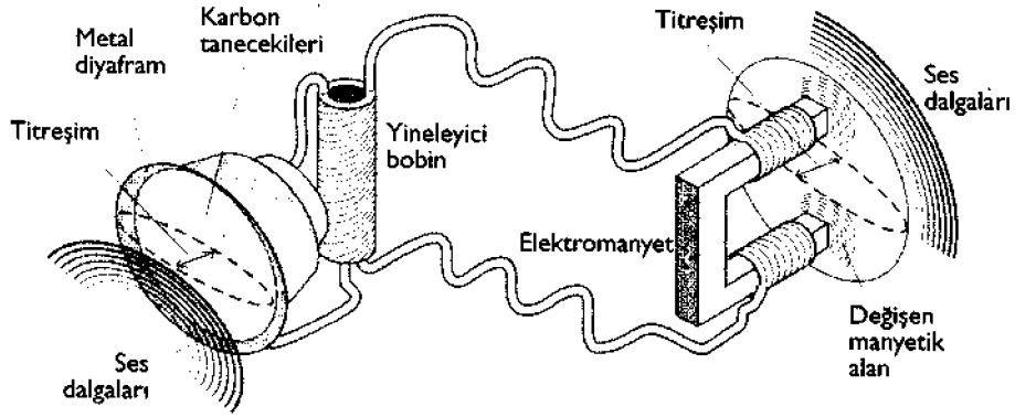
Resim 6-8. ELEKTRİK Lİ SES AKTARIMI, Telefon ses enerjisini elektrik enerjisine çevirmenin ve daha sonra da tersini yapmanın en basit aygıtıdır ama burada tanımlanan ilke bütün ses aktarımlarının temelidir. Buradaki anahtar kavramlar ses dalgalarını elektrik dalgalarına çeviren mikrofona (ya da ağızlığın) karbon taneceklerinden oluşması, amplifikatör olarak işleyen yineleyici bobin -basit bir dönüştürücü- ve elektrik sinyalini tekrar sese çeviren hoparlörün (ya da kulaklığın) elektromanyet-diyafram kombinasyonudur.
