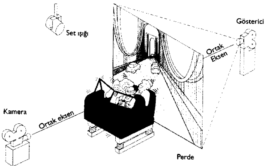
Resim 2-57. ARKADAN GÖSTERİM. Kamera ve gösterici, aynı anda çalışmaları için ayarlanır, böylece kameranın çekim yaptığı aynı anda gösterici de bir çerçeveyi yansıtır. Sahnenin önündeki dekor arabada eğlenen oyuncular, arkalarındaki yarı saydam perdenin yansıtmayacağı biçimde aydınlatılır, bu yarı saydam perde yalnızca göstericiden gelen ışığı geçirir. Arabanın yol aldığı yansımasını yaratmak için alt tarafa yerleştirilen yaylara dikkat edin.
