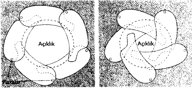
Resim 2-15. DİYAFRAM. Fotoğrafik sistemin en basit olduğu kadar en önemli öğelerinden biri olan diyafram genellikle beş ya da altı tane birbirine geçmiş ince yaylı metal plakadan oluşur. Bunlar açıklık ölçüsünün kolayca düzenlenebilmesi için birbirlerinin üzerine biner.
