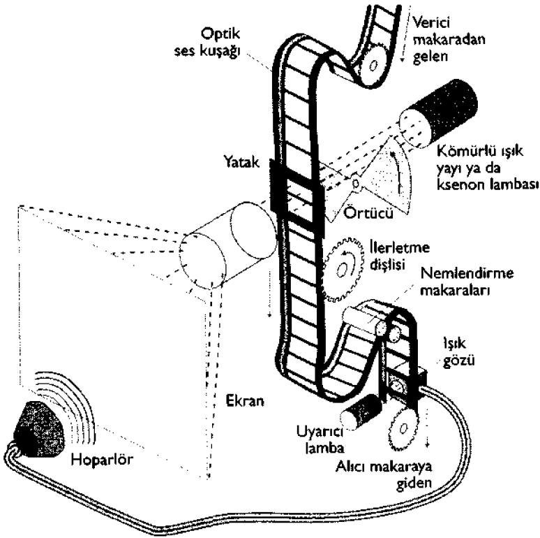
Resim 2-64. STANDART GÖSTERİCİ. Daha küçük dişliler filmi verici makaradan alıcı makaraya doğru iter. Ana dişli filmi aralıklı olarak ilerletir. Bu işlem Malta haçı dişlisiyle ilişkilidir (bak. Resim 2-21). Ses kuşağının sürekli ve pürüzsüz olarak okunabilmesi için bir dizi makara, ses kafasına varmadan önce filmin aralıklı hareketini yavaşlatır.
