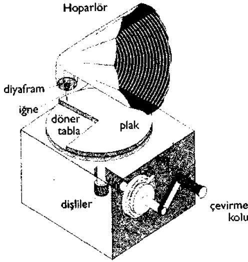
Resim 6-6. MEKANİK GRAMOFON. Çevirme kolu enerjiyi sağlar, ana yay depolar ve dişliler de aktarır. Plakin oyukları sinyali depolar, iğne aktarır, diyafram bunu mekanik titreşimden ses sinyaline çevirir, hoparlör sesi yükseltir.
