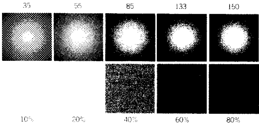
Resim 6-2. YARIMTON EKRANLAR. İnce başına 35 satır ile ince başına 55 satır ekranlar özel efektler hariç, her şey için fazlasıyla kaba ekranlardır. 85 satır ekran gazeteler için standarttır. 133 satır ekran en çok kitaplar için kullanılır. (Bu kitapta 133 satır ekran kullanıldı.) İnce başına 150 satır ekran, en iyi ayrıntıların esas olduğu -tıbbi illüstrasyonlar gibi- özel uygulamalarda kullanılır.
