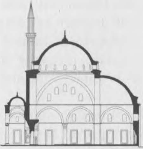
Eski Fatih Camisi'nin kesit restitüsyonu.
