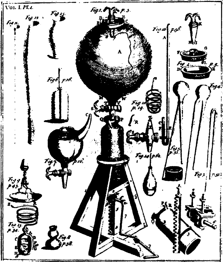
Şekil 21- Robert Boyle'un ilk hava pompası. Kaynak: Robert Boyle, New Experiments Physico-mechanical Touching the Sp- ring of the Air (1660).
