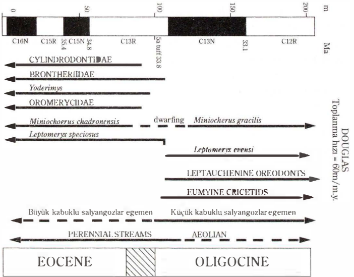
Şekil 14. Eosen-Oligosen geçişindeki (33-34 milyon yıl önce) evrimci yapılar, Wyoming Douglas yakınındaki katmanlarda kayıtlıydı. En üstteki manyetik kutup zaman ölçeğidir. Ortadakiler iklimsel değişiklikteki tür ve aile dizileridir. Bir çoğu arkasından hızlı bir türleşme ve soyun tükenmesi gelen, uzayan dönemler göstermektedir. Tüm diğer memeliler (gösterilmemiştir) zaman aralığında hiçbir değişiklik göstermemektedir. Altta bağımsız olarak bir çok memeli bu iklim değişikliğini izlemese bile, bu zamanda önemli bir soğuma olayının olduğunu gösteren iklim değişikliği göstergeleri vardır.
