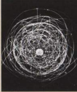
92 elektron ve 143 protonlu uranyum atomu kolayca parçalanarak büyük miktarda enerji açığa çıkarabilir.
