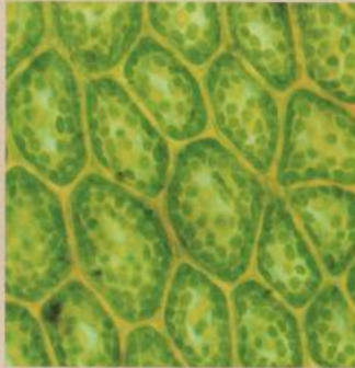
Ortalama bir yeşil bitkinin yaprağında, resimdeki hücre içi küçük noktacıklar gibi, beş milyar kloroplast bulunur.
