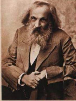
Dmitri Mendeleyev'in periyodik tablosu 1871'de şüpheyle karşılandı.
