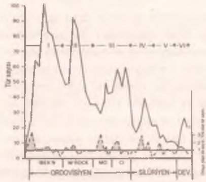
Ordovisiyen-Silüriyen devirlerinde Konodont evrimi.
