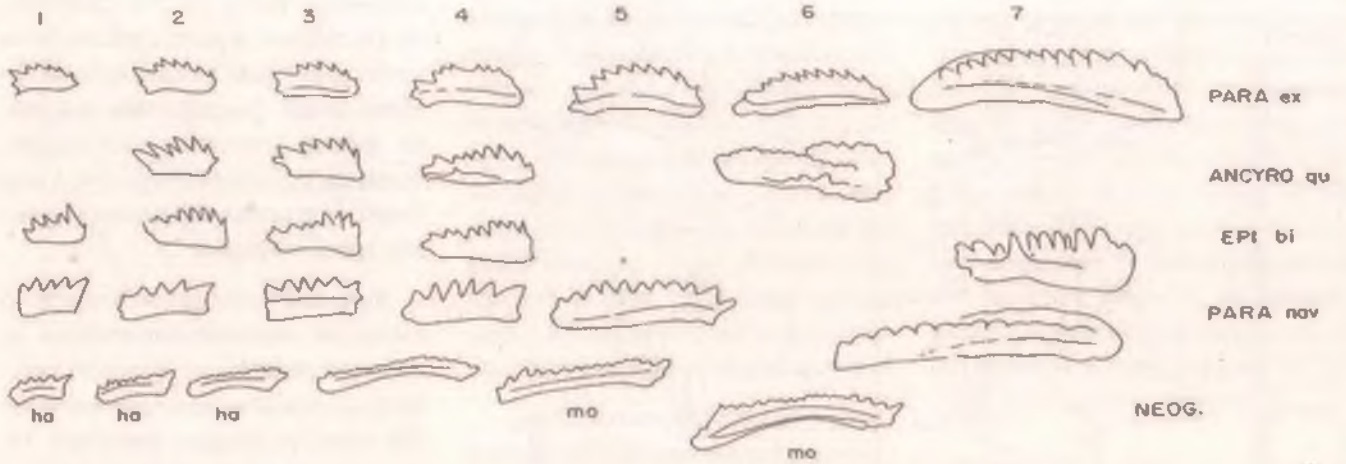
Neogondolellinae'nin ontojenisi ve evrimi 1-3 erken ontojenik "neospathid" evre 4-7 çeşitli adult evreler PARA ex: paragondolella excelsa ANCYRO qu: Ancyrogondolella quadrata EPI bi: Epigondolella bidentata NEOG mo: Neogondolella mombergensis NEOG ha: N. Haslachensis-watznaueri
