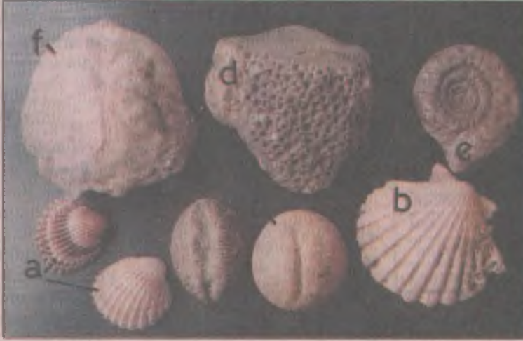
Lamelli branchiata'lardan Cardium (a) ve Pecten (b), tek yaşayan mercanlardan Cyclolites (c), masif koloni halinde yaşayan mercanlardan Hexagonaria (d), kafadan bacaklılardan Ammonit lerin güzel örneği Lithoceras (e), deniz kestanelerinden Clypeaster (f) örnekleri.
