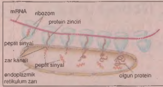
Şekil 1: "Sinyal hipotezi". Hücre DNA'sında taşınan genetik şifre, protein sentezine katılan m-RNA aracılığıyla aktarılır. Sentez edilen proteinin üzerinde taşıdığı "sinyal" bir aminoasit zincir parçasıdır. Bu sinyal sayesinde protein endoplazmik retikulum zarı üzerindeki kanallarda yolunu bulur. Protein sentezi endoplazmik retikulum içinde sonuçlanır ve protein daha sonra yine üzerindeki sinyalin yönlendirmesiyle hücre dışına taşınır.
