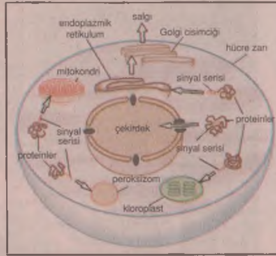
Şekil 2: Yön gösteren sinyallerle protein ulaşımının kontrolü. Şekildeki kloroplast yalnızca bitki hücrelerinde mevcuttur. Yeni sentezlenen protein üzerindeki adres kodlarıyla hücre içinde gideceği doğru yeri bulur. Bu posta kodu proteinin bir parçasıdır, genellikle proteinin uç kısmında yer alır.
