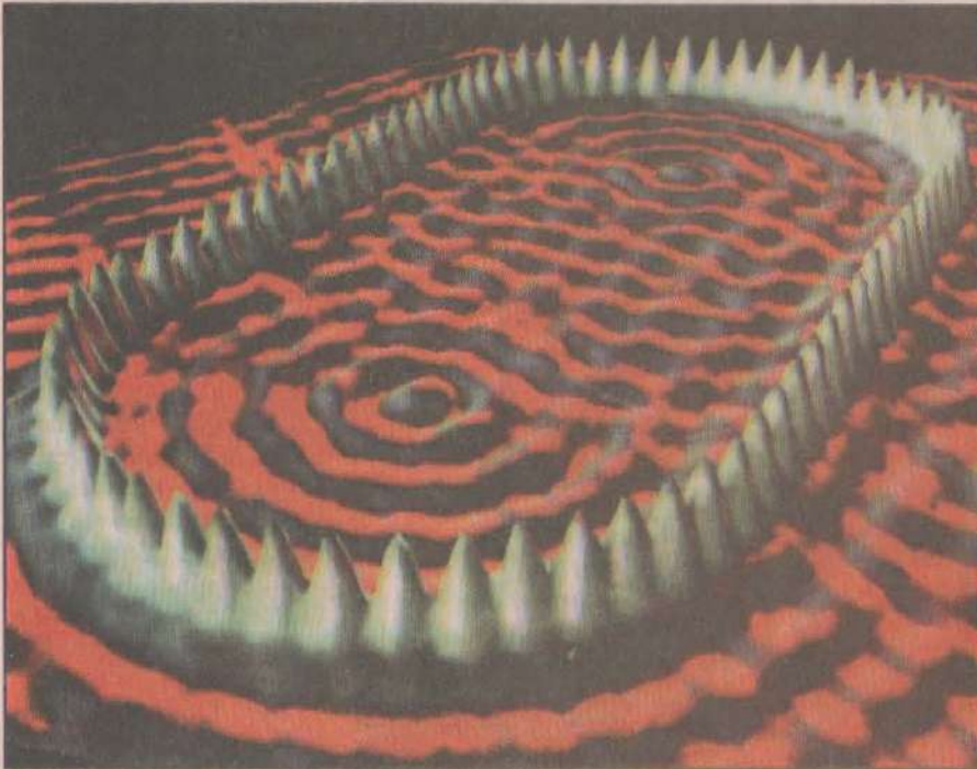
Kuvantlık hipodrom: Taramalı tünelleme mikroskobu, atomları hem "görmek" hem de kontrol etmek için, kuvantal ilkeleri kullanır. Burada, yarış alanı şeklinde dağılmış mavi koniller demir atomlarıdır. Dalgalanmalar atomların salınımlarıyla gerçekleşiyor.
