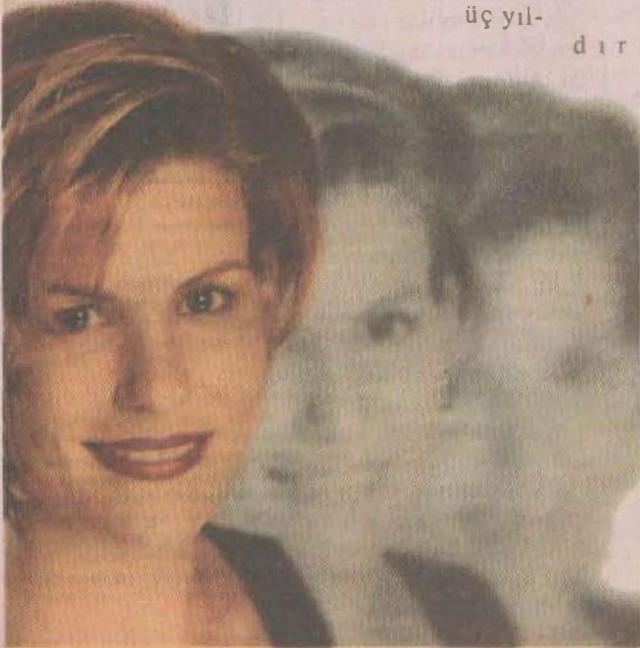
Deney çift gördüğünde: Resimdeki atom, kuantal çoğulluk sırasında "suçüstü yakalandı"; aynı anda iki ayrı konumda gözlemlendi. Bu kuantal "heryerdellik" ilk defa 1996 yılında Colorado'daki National Institute of Standards and Technology'de gerçekleştirildi.
