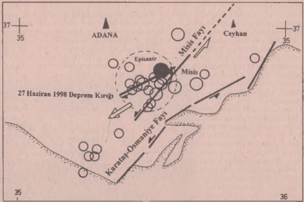
Şekil 2. 27 Haziran 1998 depremine neden olan fay ve civarında yer alan diğer fayların dağılımını gösteren harita
