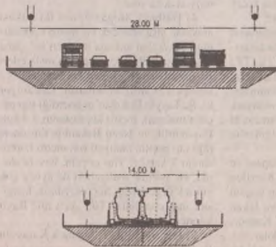
Üstte karayolu köprüsünün, altta metro köprüsünün en kesitleri
