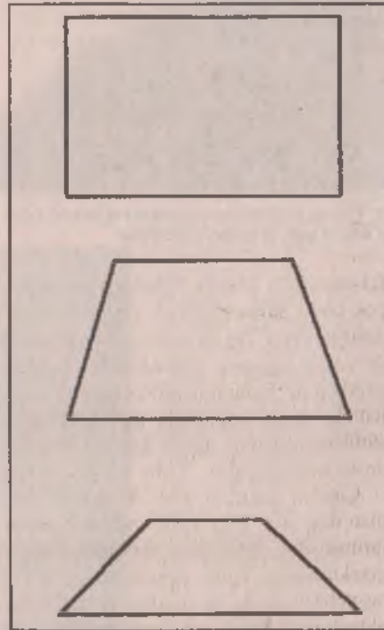
Şekil-1 Bir dikdörtgenin retina gibi bir yüzeye yansıması, yansıma açısına bağlı olarak farklı şekillerde olur.
