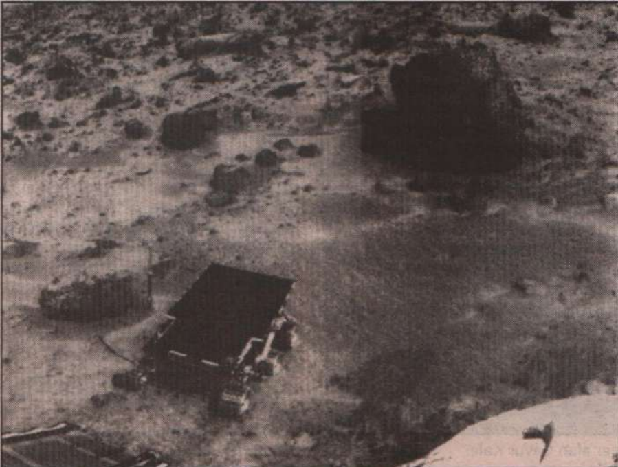
Sojourner "Yogi taşı"na doğru yol alırken. Ücretsiz PDF Kitap Arşivi - https://rante.org "Yogi taşı"nı incelerken sıkışıyor ve bir süre hareket ettirilemiyor.
