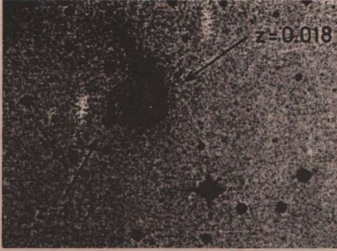
Şekil 7 a. Gökadaya ışıklı bir köprüyle bağlanan PKS 1327-206 kuazarı
