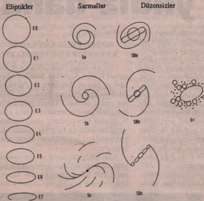
Şekil 1. Gökadaların Hubble sınıflaması. E ve S türleri arasındaki geçiş türü SO'dur. a, b, c, (d, m) dizisiyle gösterilen gökadalardan sarmal kolları disk çevresinde sıkı sıkıya sarılı ve iyi tanımlanmış kollardan açık, parçalanmış kollara doğru gidişi anlatılır.
