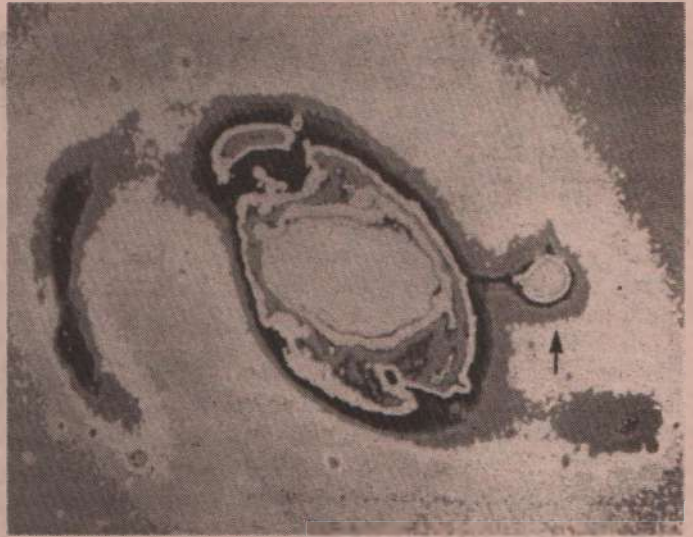
Şekil 5. NGC 4319 sarmal kollu gökadası ve okla gösterilen Markarian 205 kuazarı.
