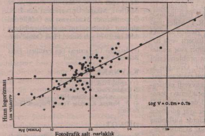
Şekil 2. Fotoğrafik salt parlaklığa karşı hızın logaritmasını gösteren Hubble ilişkisi. Her bir nokta bir gökadayı temsil etmektedir.
