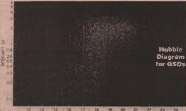
Şekil 4. Kuazarlar için çizilmiş olan görünürdeki parlaklık-kırmızıya kayma bağlantısı. Grafikte 7315 kuazar yer almaktadır.
