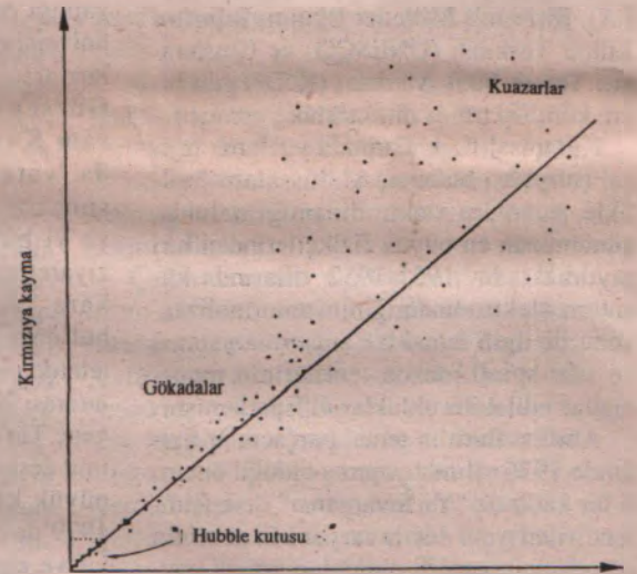
Şekil 3. Hubble kutusu dışındaki bazı gökadalardan ve kuazarlardan doğrusal bağıntıyla temsil edilemez. Bu nedenle de evrenin genişlemesinden söz edilemez!
