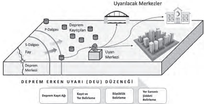
Şekil 2. Deprem Erken Uyarı (DEU) düzeneğinin şematik gösterimi. Deprem olur olmaz P dalgası daha hızlı olduğundan S dalgasından daha önce ulaşır. Kayıtçıların kayıtlarını toplayan uyarı merkezi veriyi işleyip depremin yerine, büyüklüğüne ve ulaşacağı yerlerdeki sarsıntı şiddetine (ivme) karar verir ve ilgili noktalara iletir.
