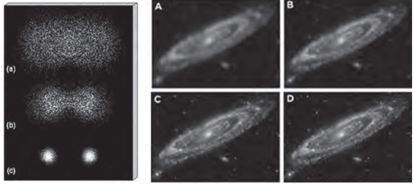
Açısal çözünürlük: (sol) açısal çözünürlüğün artmasıyla bulutsu izlenimi veren ortamın aslında çift yıldız dizgesi olduğu anlaşıyor. (sağ) Bir gökadanın görüntüsünde açısal çözünürlük A-B-C-D sırasıyla görüntüde netliği sağlıyor.
