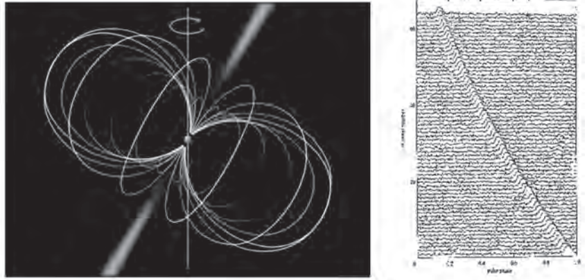
Zaman çözünürlüğü: (sol) Bir atarca modeli. Özetteki nokta nötron yıldızı; beyaz çember yay parçaları manyetik alan kuvvet çizgileri; gri renkli beysbol sopası benzeri bölgeler nötron yıldızın manyetik uçlak bölgelerinde üretilen radyo dalgaları. Nötron yıldızın dönme dönemi saniyenin fraksiyonlarındadır; (sağ) Atarcadan gözlemciye ardışık olarak gelen değişik frekanslardaki ‘deniz feneri benzeri patlamalar’. Zaman çözünürlüğü bu denli gelişmeden önce atarcadan algılanan radyo dalgaları sürekliymiş izlenimi veriyordu.
