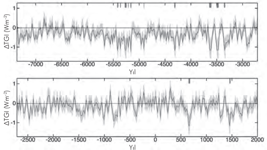
Şekil 3: Son 9300 yıl için, ^{10}\text{Be} izotoplarının buzullar içinden elde edilmiş zaman serisi kullanılarak elde edilmiş toplam güneş ışımasını (TGI) miktarı grafiği 2 . Grafikte TGI'nin 1986 yılındaki değerine göre sapma miktarları negatif ve pozitif değerler olarak verilmiştir.
