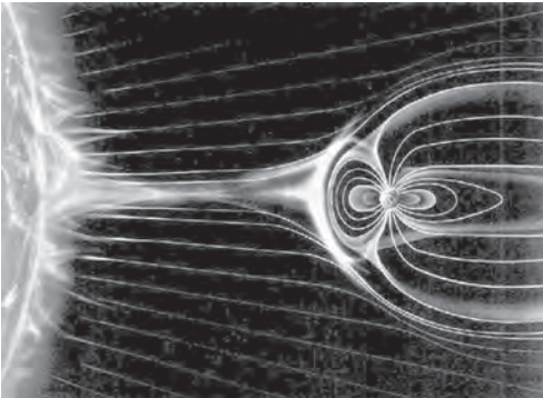
Şekil 2: Çizimde solda Güneş ve Güneş'in açık manyetik alan çizgileri sağda ise Yer ve manyetik alan çizgileri görülüyor. Güneş'in açık manyetik alanı Yer'i kozmik parçacıklardan büyük oranda korumaktadır.
