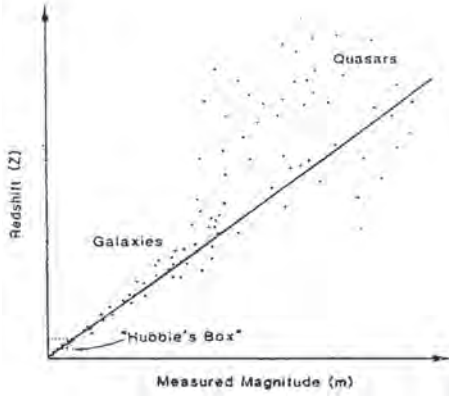
Şekil 3. Hubble kutusu ("Hubble's Box") dışındaki bazı gökadarlar ve kuazarlar doğrusal bağıntı ile betimlenemez. Bu nedenle evrenin genişlemesinden söz etmek doğru değildir.
