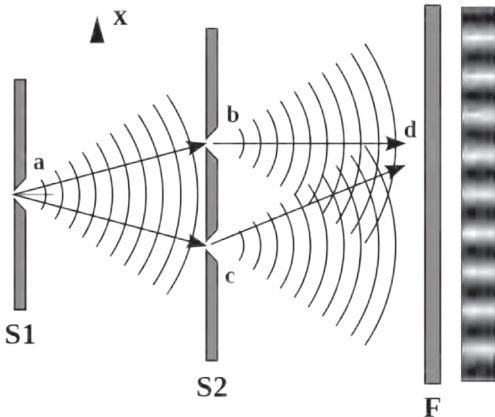
Resim 3: Genel bir Young deneyi tasviri. Bu deney tasarım şeması, dünyadaki hemen tüm fizik bölümlerinde standart olarak kullanılır. Kaynak: ODTÜ Optik Deneyleri Dersi Rapor Kitabı.
