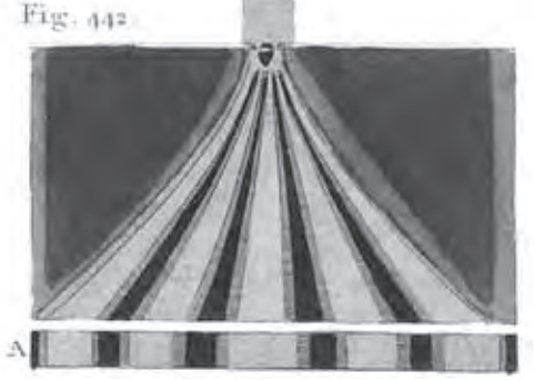
Resim 2: Young'ın kendi çizimiyle çift yarık deneyi. 1807'de ışığın dalga kuramını anlattığı ders kitabından alınan çizim, tarihteki ilk çift yarık deneyi tasviridir.
