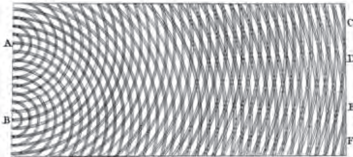
Resim 1: Thomas Young'ın fizik notlarından kendi çizimiyle girişim desenleri. A ve B noktalarından dalgalar yaratılmaya başlanırsa C, D, E ve F noktalarında yıkıcı girişim desenleri gözlenecektir.
