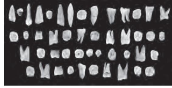
Çin'in Hunan eyaleti Daoxian'ın bir mağarasındaki kazılar sonucunda bulunan düzinelerce diş fosili günümüzden 80-120 binyıl öncesine tarihleniyor ve modern insana ait olduğu düşünülüyor.
