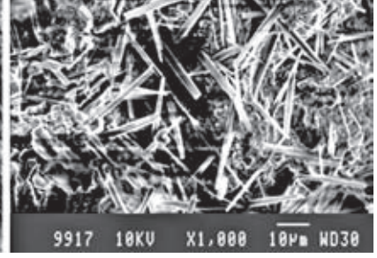
Eriyonit mineralleri içeren pomza parçalı volkanik tüf kayası (Tuzköy-Gölşehir) ve eriyonit mineral iğneciklerinin taramalı elektron mikroskop (SEM) görüntüsü
