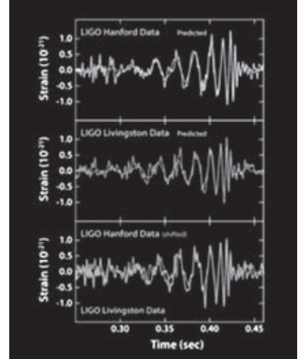
LIGO merkezleri tarafından yakalanan sinyaller (Kaynak: ligo.caltech.edu).
