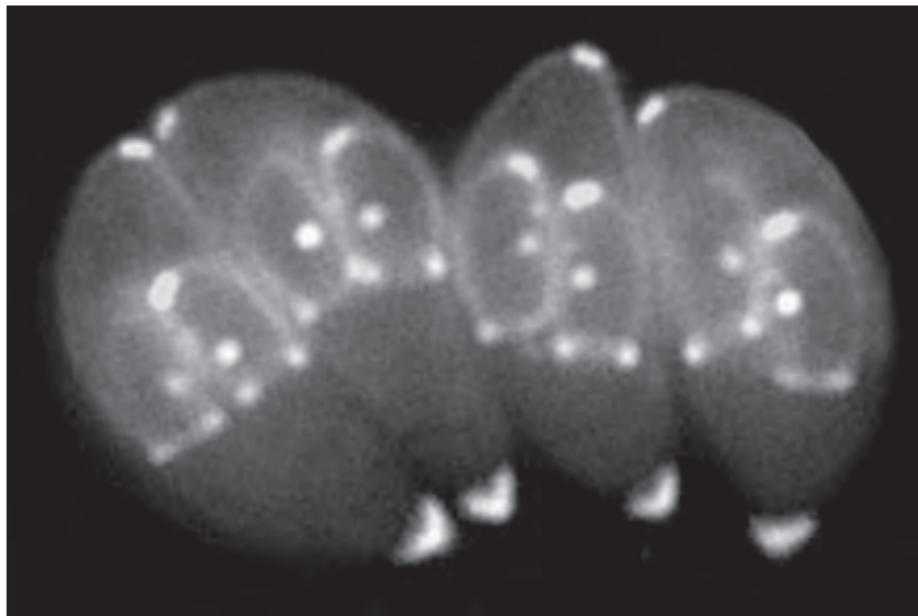
Toxoplazma gondii bölünürken...
