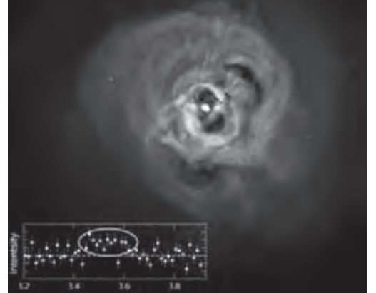
3,55 keV'lik ışıma ve Perseus kümesi.
