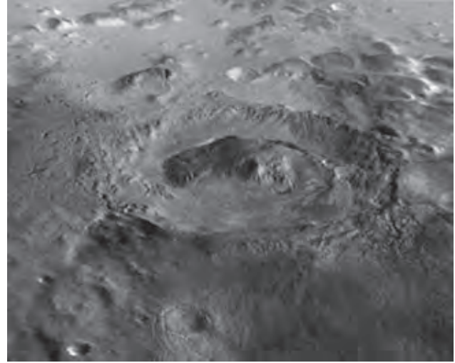
Mars'ta su bulunduğuna dair kanıtlar içeren Gale Krateri.
