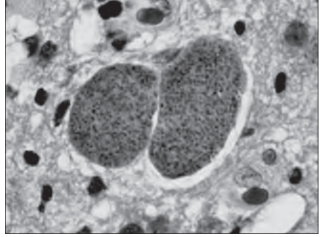
Ara konağın beyinde oluşmuş T. gondii doku kistleri.
