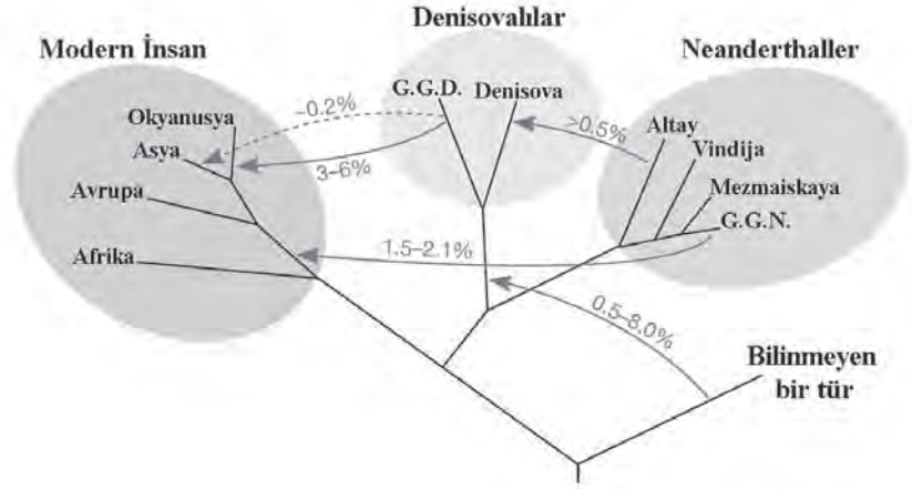
Şekil 2: Geç Pleyistosen dönem boyunca muhtemel gen akışlarının modeli. Bu modelde Neandertaller ile Denisovalılar ve modern insan arasındaki tahmini oranlardaki gen akışını görebilirsiniz. Ayrıca henüz bilinmeyen bir türün de Denisovalıların gen havuzuna katkıda bulunduğu saptandı.
