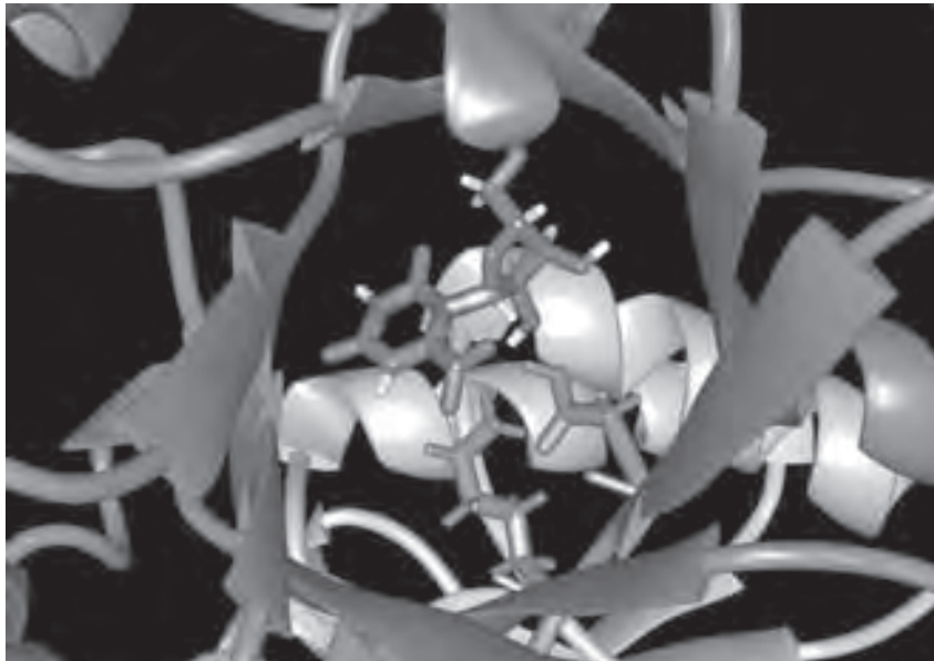
Anton yüksek hızla moleküler simülasyonlar geliştirecek.
