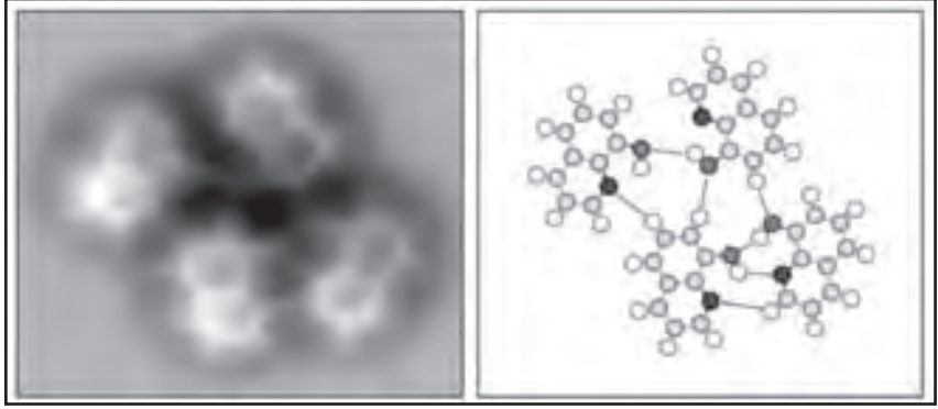
Çinli araştırmacılar ilk kez bir hidrojen bağının yüksek çözünürlüklü görüntüsünü elde etti. Solda, sağdaki modelin AFM ile elde edilmiş görüntüsü görülüyor.
