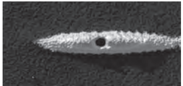
İlk lazer soğutmalı Bose-Einstein yoğunlaşması
