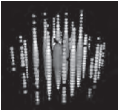
3 Ocak 2012'de tespit edilen yüksek enerjili nötrinoya ilişkin sinyaller.
