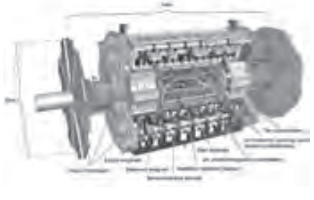
ATLAS algıcının tasarımı.
