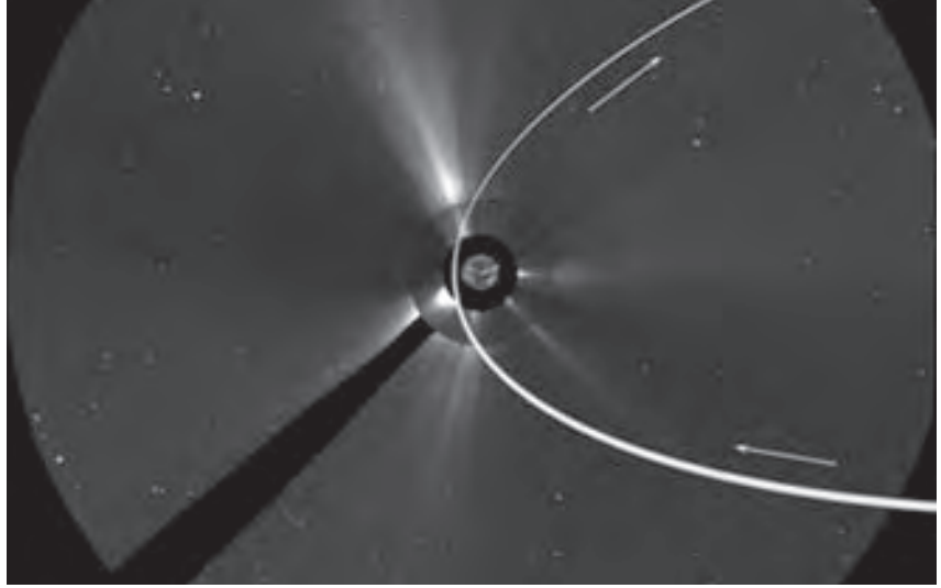
ISON kuyruklu yıldızının yörüngesi... Görüldüğü gibi Güneş'e yakın bir hiperbol oluşturacak ve 28 Kasım tarihinde en parlak, başka bir deyişle Güneş'e en yakın konumuna gelecek.
