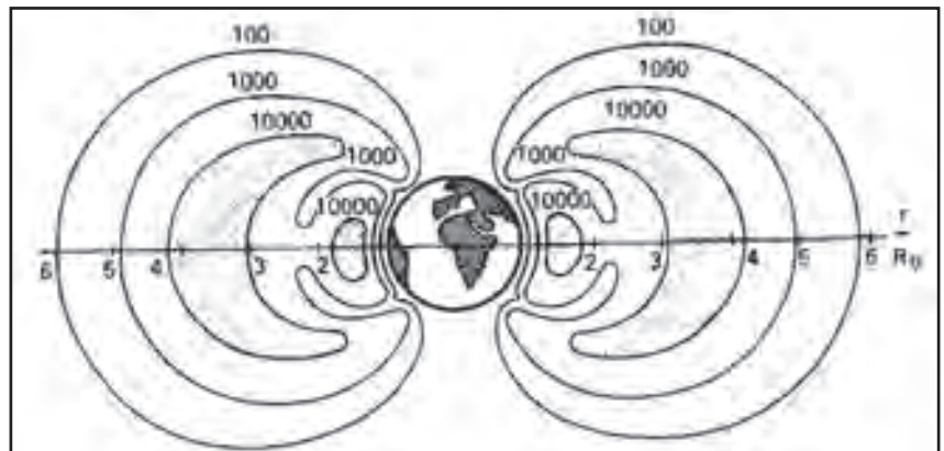
Şekil 3. Taralı bölgeler Yer'in doğal ışınlam kuşaklarını simgeler. Rakamlar kozmik ışın yeghnlık oranlarını vermektedir (L.A. Artsimovich & S.Yu Lukyanov, 1980).
