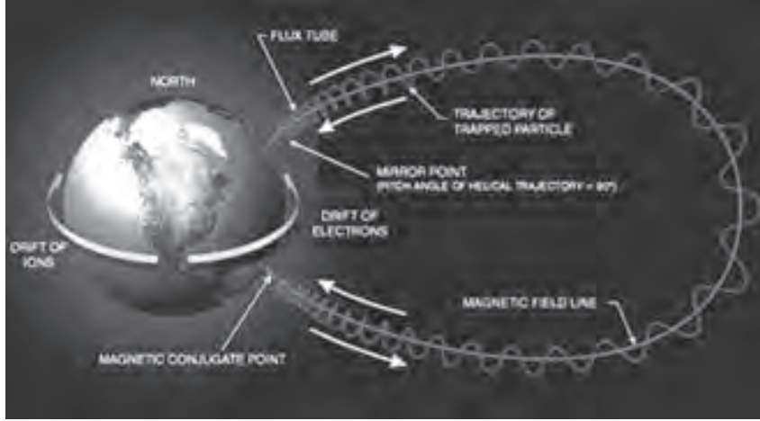
Şekil 2. Elips görünümündeki çizgi, Yer'in manyetik alan kuvvet çizgilerinden birini; sarmal yörüngeyse manyetik alan kuvvet çizgisine tuzaklanmış olan bir elektrik yüklü parçacığın yörüngesini simgeler. Tuzaklanmış olan parçacığın 3 dönemsel devinimi vardır: a) Manyetik alan kuvvet çizgileri çevresinde dolanma devinimi, b) Yer'e yakın bölgelerdeki manyetik aynalar arasında zıplama devinimi ve c) Yer'in çevresinde doğudan batıya (pozitif elektrik yüklü parçacıklar) veya batıdan doğuya (negatif elektrik yüklü parçacıklar) sürüklenme devinimi.
