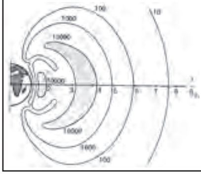
Şekil 4. Nükleer bomba patlamasıyla oluşturulan "yapay ışınım kuşağı", iç ve dış ışınım kuşakları arasında yer alıyor.
