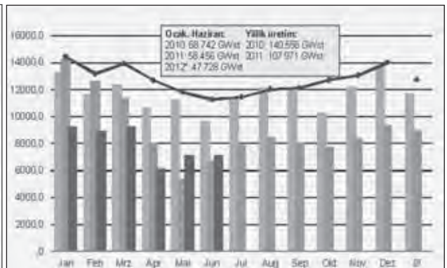
Grafik 2. Almanya'da nükleer santrallerden 2010, 2011 ve 2012'de aylara göre üretilen elektrik enerjisi (GigaWatt-saat).
