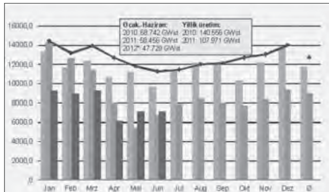
Grafik 1. Almanya'da fotovoltikten 2011 yılında ve 2012'nin ilk beş ayında, aylara göre üretilen elektrik enerjisi
