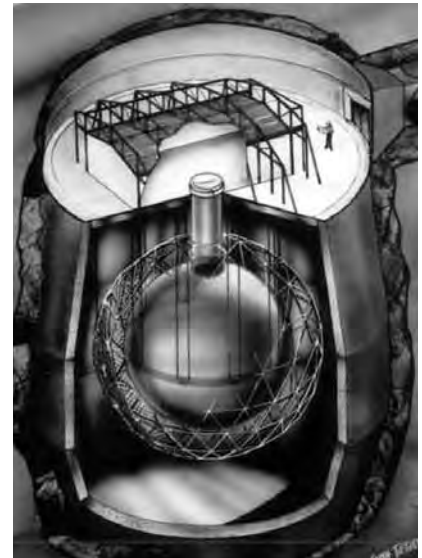
Sudbury Nötrino Gözlemevi'ndeki dedektörün tam bir betimi.
