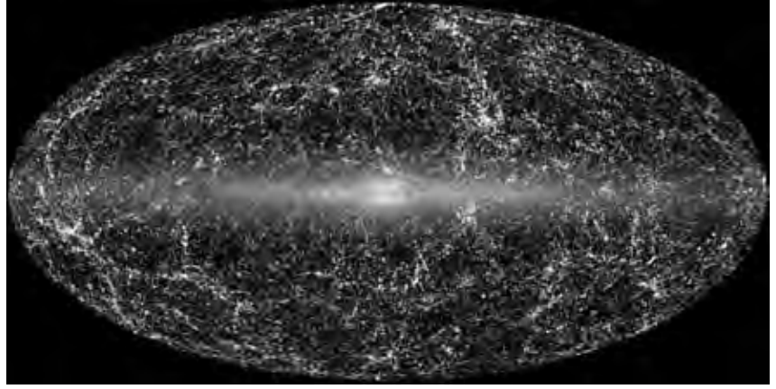
WMAP'ın taşıdığı aygıtların mikrodalga ışımasındaki sıcaklık değişimlerine dayanarak çıkarttığı Evren haritası sayesinde Evren'in yalnızca yaşına değil, genişleme hızına hatta temel içeriklerine ilişkin de oldukça duyarlı veriler elde edilmiştir.
