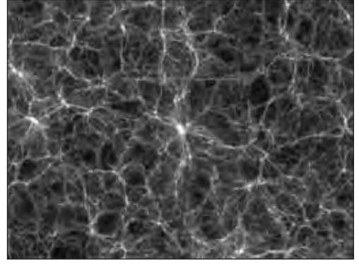
Max Planck Astrofizik Enstitüsü'nün bilgisayar canlandırmasında birkaç milyar ışık yılılık bir ölçeğe milyonlarca gökada kümesi ve süper küme ipliksi bir yapıda -sanki birbirine bağlanmış gibi- görülüyor. Gökadalardan oluşan ipliksi dokunun arasında engin boşluklar vardır.
