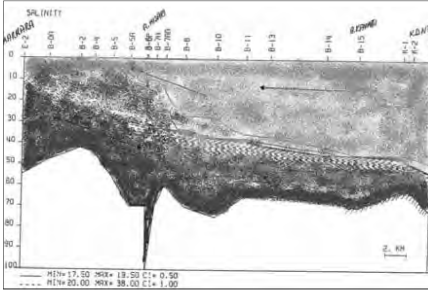
Boğaz'da akıntılar: Tam bir ikili akış sistemi. Karadeniz'den Marmara'ya gelmekte incelen su, tersini Marmara'dan Karadeniz'e giderken de yapmakta. Karışımlar en derin yerde ve Üsküdar-Beşiktaş arasında.
