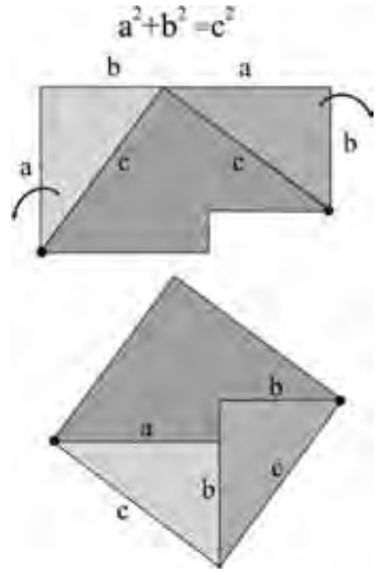
Şekil 5: İlk menteşeli parçalama
