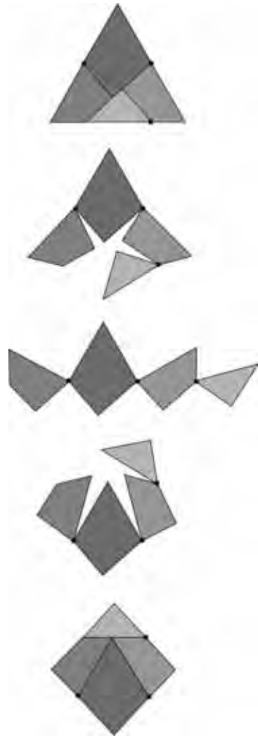
Şekil 4: Dudeney’in eşkenar üçgenden kareye menteşeli parçalaması
