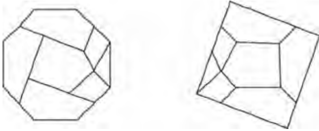
Şekil 7.1: Sekizgenden kareye bir menteşeli parçalama
