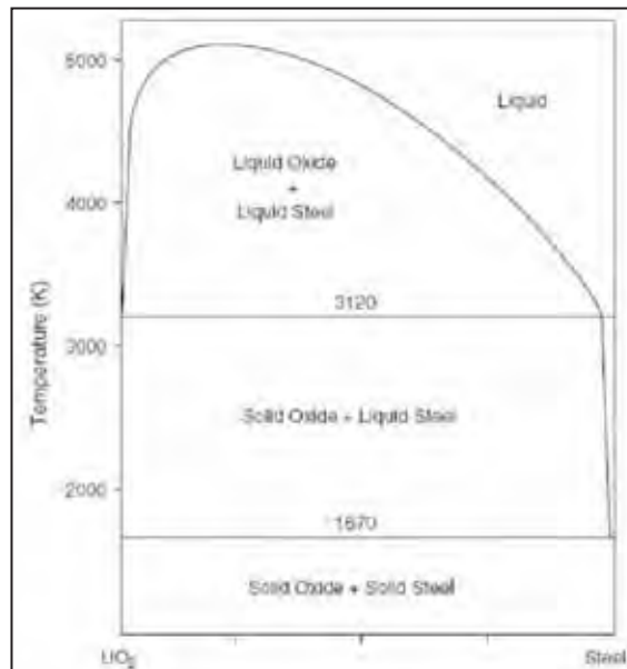
Şekilde UO_2 -Fe dizgesinin evre çizgesi (Schuiling, 2006).
