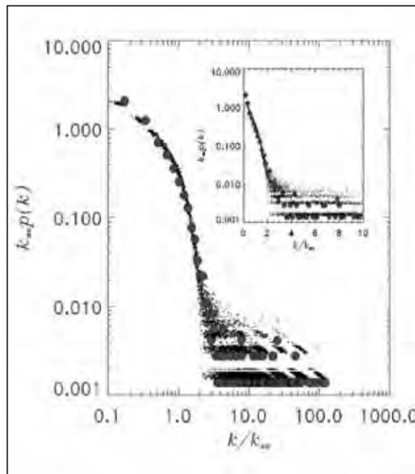
Şekil 3. Şekilde büyük noktalar bira mayasının, arkadaki küçük dağınık noktalar, model şebekesinin yüz gerçekleşiminin verilerini göstermektedirler. Yatay eksen etkileşim sayıları, ortalama etkileşim sayısına bölünmüş olarak verilmektedir. Dikey eksen ise, bu sayıda etkileşime sahip olma olasılığı, yine ortalama etkileşim sayısı ile çarpılmıştır. Eksenler logaritmiktir. Küçük şekilde ise, yatay eksen doğrusal seçilerek, eğrinin başlangıç kısmının üstel bir ifadeye uyduğu gösterilmiştir.
