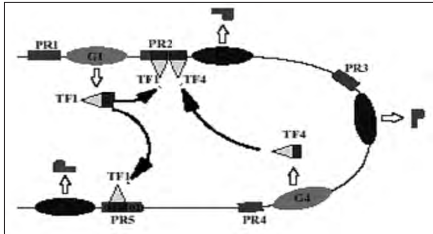
Şekil 2. Bir kromozom üzerinde gen düzenleme şebekesinin şematik gösterimi (25). Genlerin (G1, G2,...) ürettikleri proteinlerden bazılarının (TF1, TF2,...) üçgenlerle işaretlenmiş rasgele "bağlanma dizileri" atanmıştır. Eğer başka genlerin bitişindeki, kendileri de rasgele seçilmiş olan, "düzenleme bölgeleri" (PR1, PR2,...) içinde bu bağlanma dizileri mevcutsa, bu proteinler oraya bağlanarak ilgili geni baskılayacak ya da üretime geçmesini teşvik edeceklerdir. Örneğin şekildeki G1 geni, ürettiği TF1 proteinini aracılığı ile G2 ve G5'i düzenlemektedir. G2 ve G3'ün ürettiği proteinler (P) ise yapısal proteinler olup DNA üzerine bağlanmamaktadırlar. (Gri tonlu bu gösterimde G2, G3 ve G5 genlerinin etiketleri seçilememektedir.)
