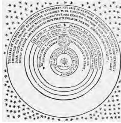
Kopernik'in Güneş merkezli evren modeli.
