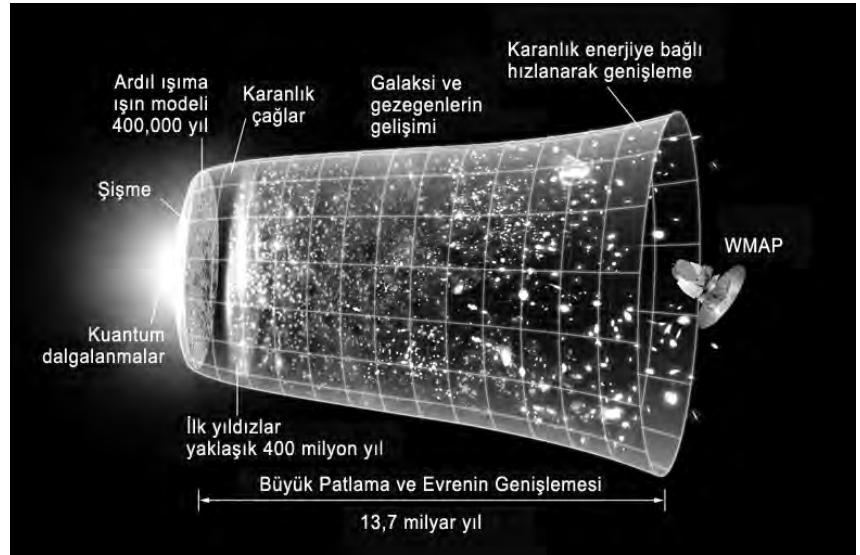
Big Bang'ın ilk döneminden günümüze kadar evrenin genişlemesinin grafik tarzındaki temsili. WMAP uydusu verileriyle 2006 yılında hazırlanmıştır.
