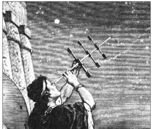
İlkçağların büyük astronomlarından Hipparchos'u betimleyen bir tablo.
