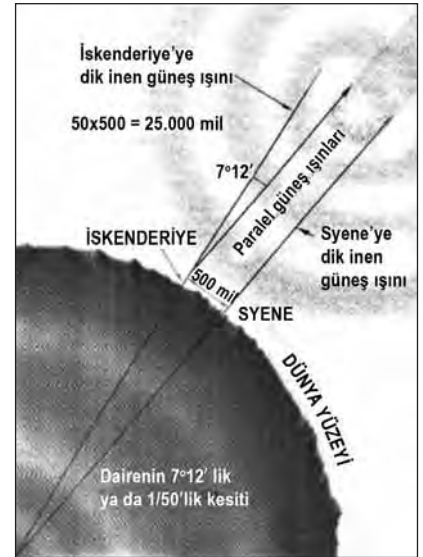
Eratosthenes'in dünyanın çevresini bulmakta kullandığı yöntem.
