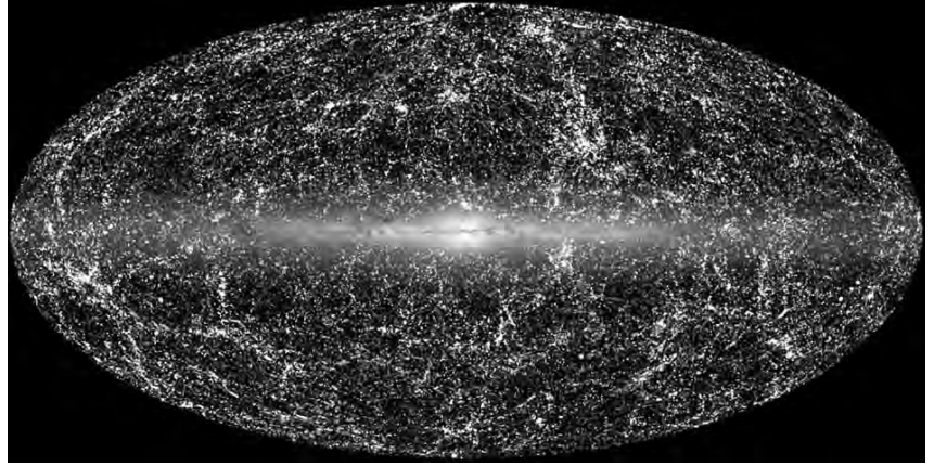
1965 yılında Büyük Patlama modelinin “köz”ü, mikrodalga ışıınımı keşfedildi. Tüm evrene dağılmış olan bu fotonlar tüm yönlere doğru yayılıyordu.
