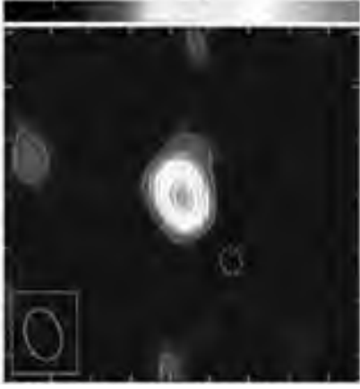
ELSEA radyoastronomi projesinde elde edilmiş bir mikrouasar görüntüsü.
