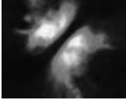
Hubble Uzay Teleskopu'nun çektiği bu fotoğrafta, disk şeklindeki, koyu bir toz ve gaz bulutunun parlayan bir yıldız iki eşit parçaya bölündüğü görülüyor. Bu tür diskler gezegen ve yörüngede dönen diğer cisimleri meydana getiren planetesimallerin oluşumu için ham madde sağlamaktadır.
