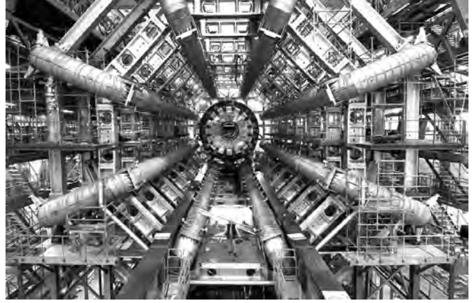
CERN'deki Büyük Hadron Çarpıştırıcısı.
