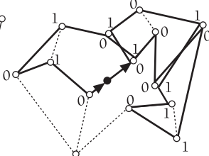
Prens saraydan ok yolunda yola çıkıyor. Önce sola (0) sapıyor. Sonra sağa (1). Tam 17 kez sol sağ yaptığımda sarayına geri dönüyor. İki defa aynı yoldan geçiyor.
