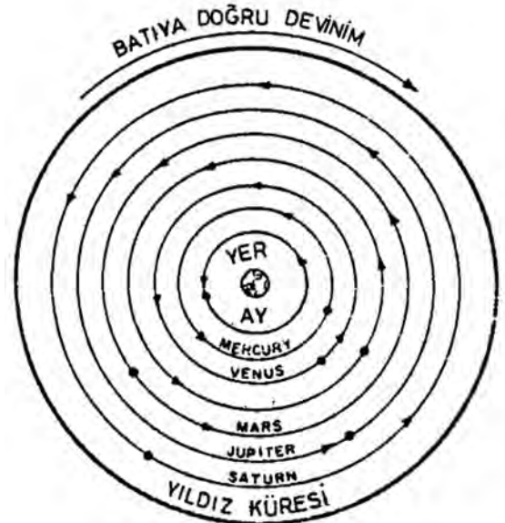
Şekil 1. İki küre evrenindeki gezegen yörüngelerinin yaklaşık biçimi. En dıştaki çember yıldız küresinin tutulum düzlemiyle arakesitidir.
