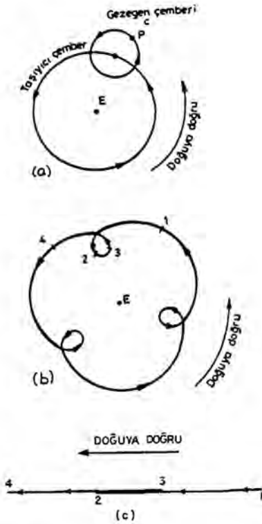
Şekil 2. Taşıyıcı çember-gezegen çemberi ikilisinin en basit biçimi (a) da gösterilmiştir. (b) gezegenlerin tutulum düzleminde gösterdikleri ilmi devinim. (c) Yer'deki (E) bir gözlemcinin devinimin 1234 konumlarını gözleyişi.
