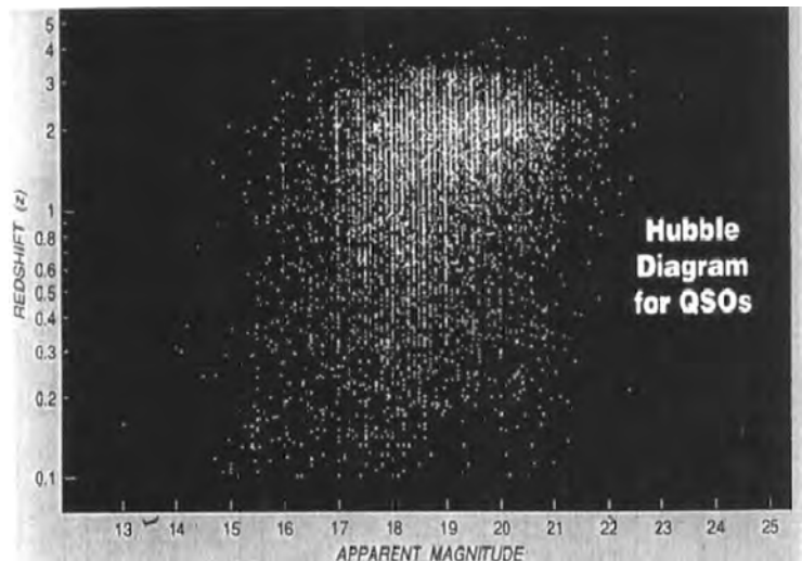
Şekil 4. Kuazarlar için Hubble Bağıntısı. Grafikteki noktaların bir doğru ile anlatılamayacağına dikkat ediniz.
