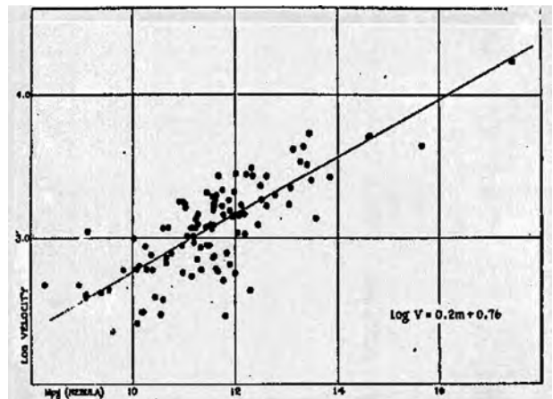
Solda şekil 1: Gökadalara Hubble sınıflaması. E ve S türleri arasındaki geçiş türü S0'dır. a, b, c, d, m dizisi ile gösterilen gökadalara sarmal kolları disk çevresinde sıkı sıkıya sarılı ve iyi tanımlanmış kollarıdan açık, parçalanmış kolları doğru gidişi anlatır. Aşağıda şekil 2. Hubble'in Sb türü gökadalara için oluşturduğu fotografik salt parlaklık-hız logaritması grafiği.
