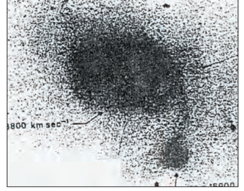
Şekil 6: NGC 7603 gökadası ve ona ışıklı köprü ile bağlanan Parkes 132-206 kuazarı.
