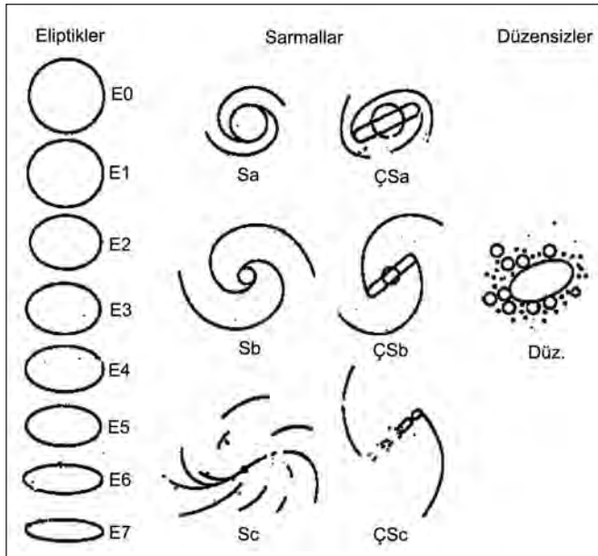
Solda şekil 1: Gökadalara Hubble sınıflaması. E ve S türleri arasındaki geçiş türü S0'dır. a, b, c, d, m dizisi ile gösterilen gökadalara sarmal kolları disk çevresinde sıkı sıkıya sarılı ve iyi tanımlanmış kollarıdan açık, parçalanmış kolları doğru gidişi anlatır. Aşağıda şekil 2. Hubble'in Sb türü gökadalara için oluşturduğu fotografik salt parlaklık-hız logaritması grafiği.
