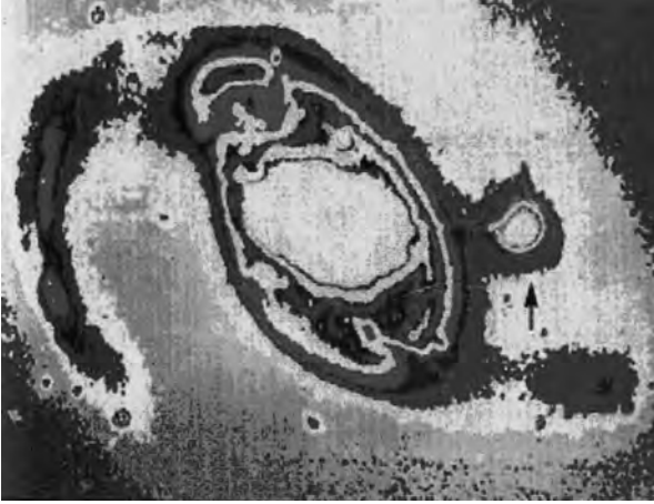
Şekil 5. NGC 4319 sarmal kollu gökadası ve hemen yanında okla gösterilen Markarian 205 kuazarı.
