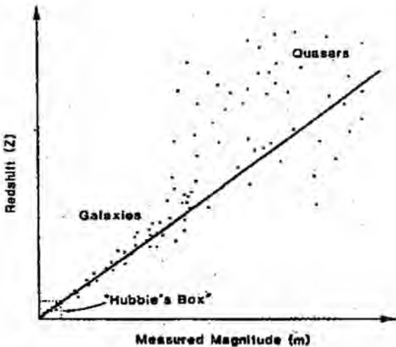
Şekil 3. Hubble Kutusu ("Hubble's Box") dışındaki bazı gökadalardır ve kuazarlar doğrusal bağıntı ile betimlenemez. Bu nedenle evrenin genişlemesinden söz etmek doğru değildir.
