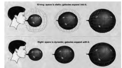
Şekil 1. Genişleyen uzay kavramına ilişkin "doğru" ve "yanlış" görüşlerin karşılaştırması.
