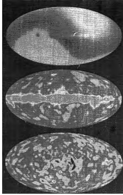
Şekil 3. COBE uydusunun çıkardığı KMAI haritası. Üst: çiftuay yönbağımlılığı. Bu yönbağımlılığın yorumu, Samanyolu’nun 600 km/s hızla Hydra-Centaurus süper kümesine doğru devindiği biçiminde yorumlanır. Orta: çiftuay yönbağımlılık etkisi haritalardan çıkarıldıktan sonra, ortadaki kırmızı şerit, Gökadamızdaki mikrodalga kaynaklarının katkısını gösteriyor. Alt: KMAI’yı “kırılten” tüm etkiler arındırıldıktan sonra KMAI haritası.
