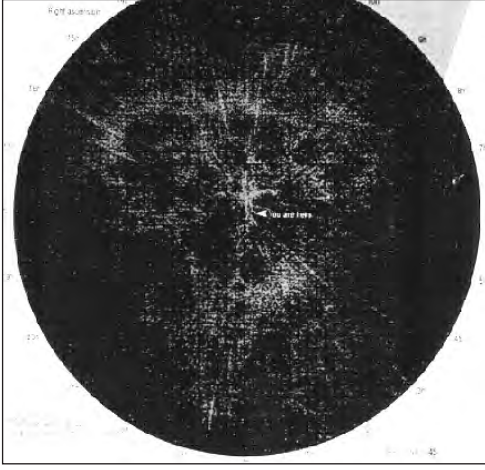
Şekil 2. Görünürdeki evrenimiz içinde bulunan gökadalara dağılımı. Samanyolu gökadası "You are here" yazılı olan özeğedir. Her bir nokta bir gökadayı simgeler. Hangi ölçeklerde alınırsa alınsın maddenin eşdağılımlı olmadığı görülüyor.
