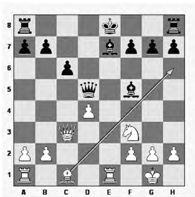
Browne-Bisguier, 1974
