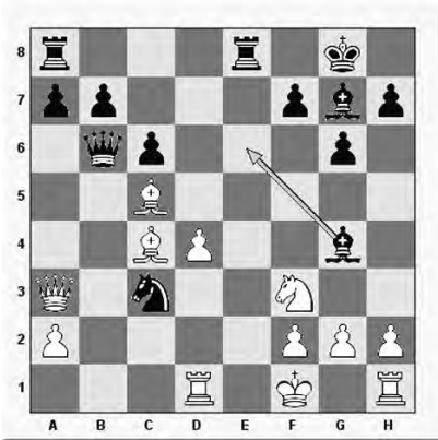
Byrne, D-Fischer, 1956
