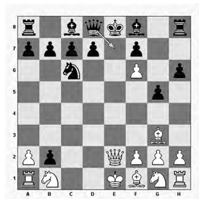
Rusakov-Verlinsky, 1947
