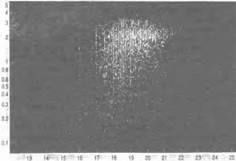
Şekil 2. Kuazarlar için Hubble ilişkisi. Kuazarları simgeleyen bu noktaları bir doğru ile temsil etmek olanaksızdır.
