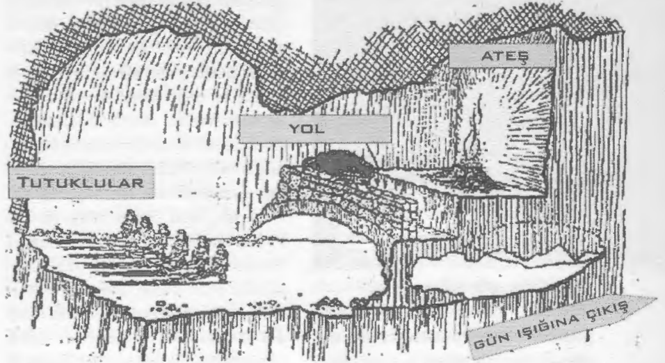
Platon'un mağarası.
