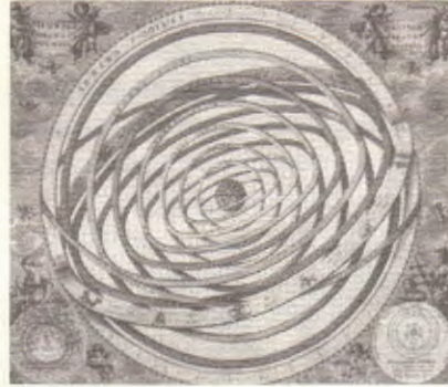
Batlamyus sistemini gösteren bir çizim.
