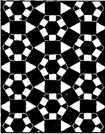
Dümorterit mineralinin kristal yapısının izdüşümü.
