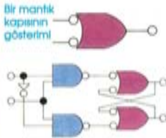
D tipi flip-flop'un şeması
