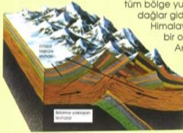
Birbirine yaklaşan iki kıtasal taşkürle levhası
